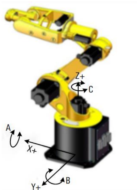
图 1-4 基础坐标系示意图
