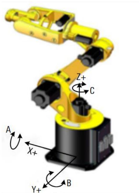
图 1-3 世界坐标系示意图
