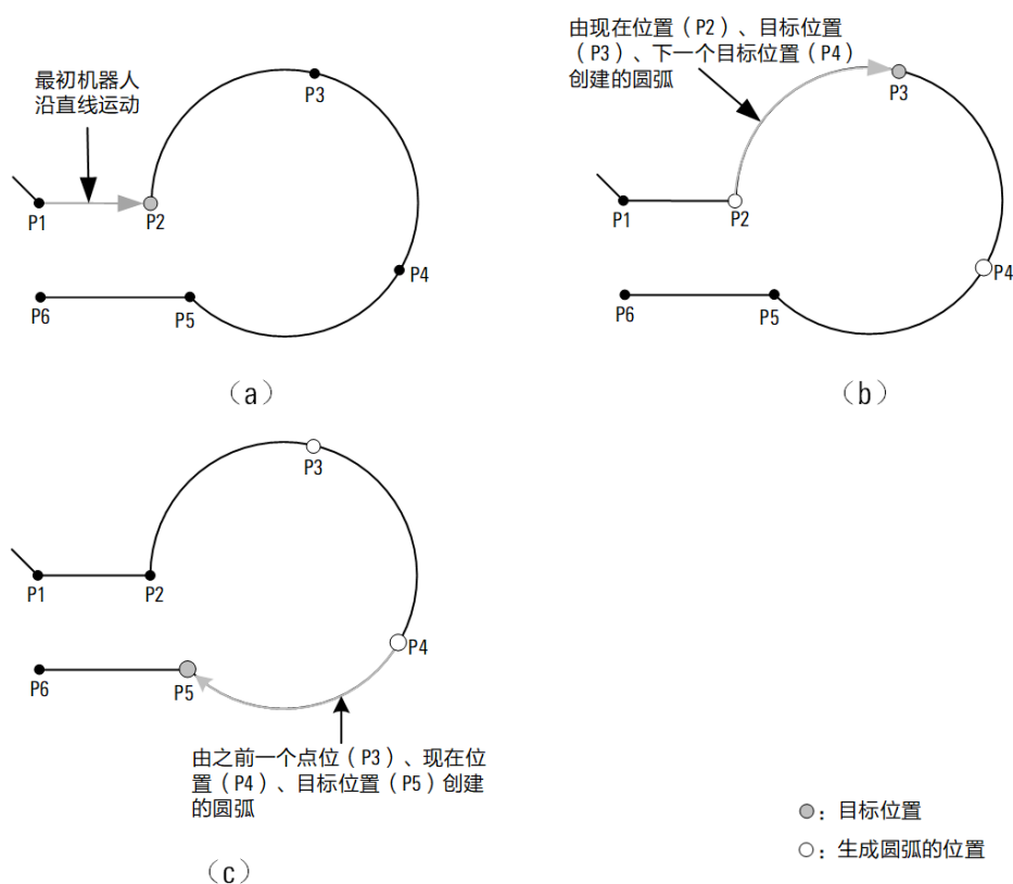
图 3-4 程序分布执行示意图
