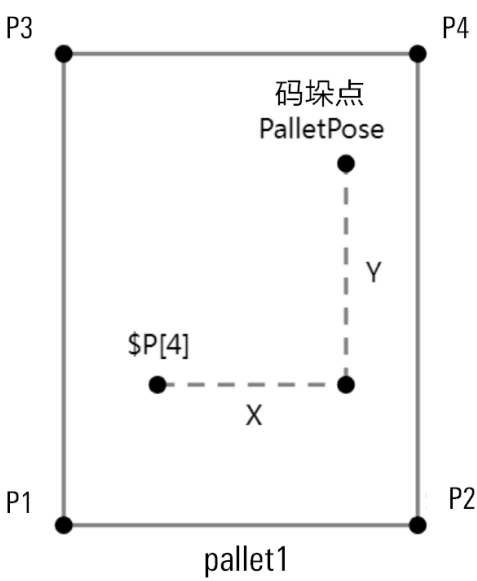
图 2-2 垛盘和码垛点示意图
